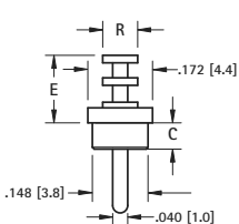
Feed-Thru
