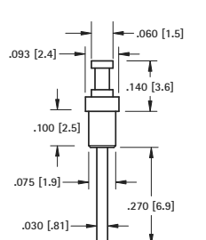
Feed-Thru
