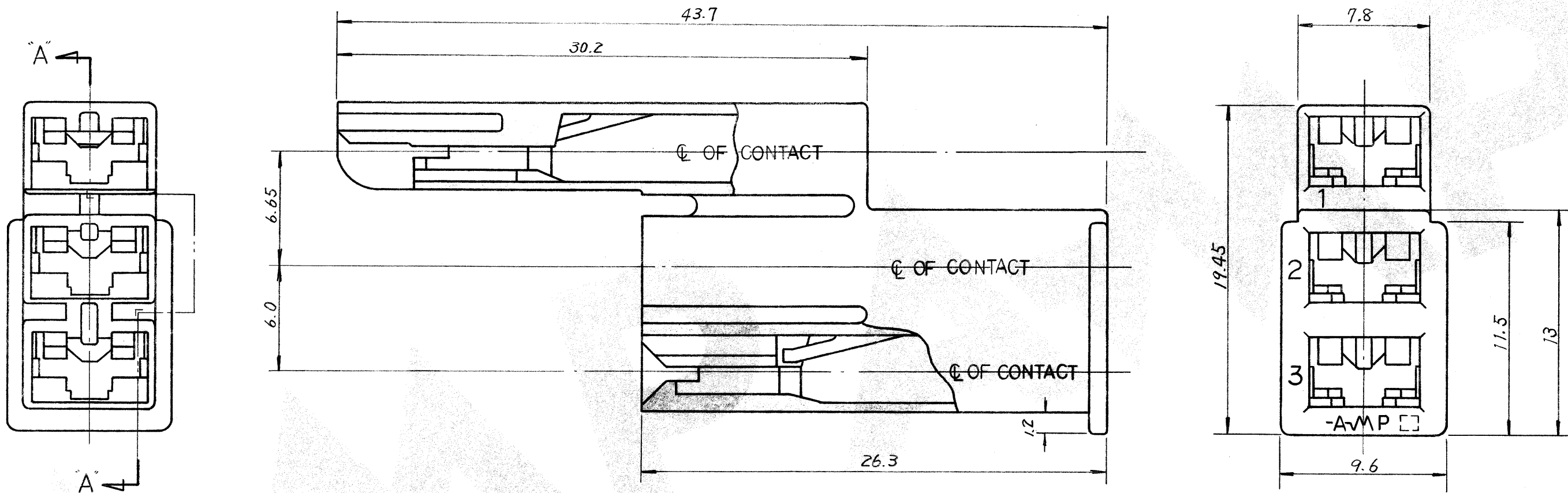
断面 "A-A"
