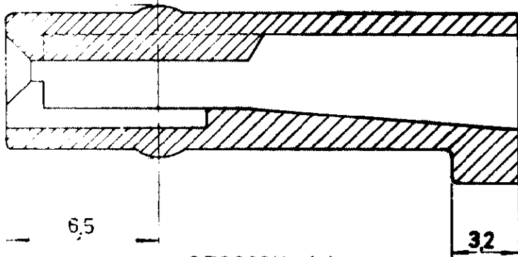
SECCION AA
