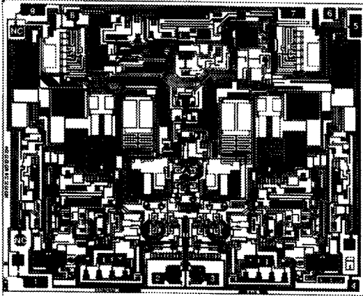
INA131 DIE TOPOGRAPHY
