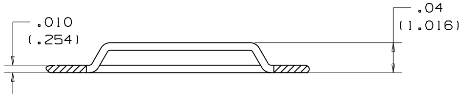
SECT "A-A" SCALE: 8x
