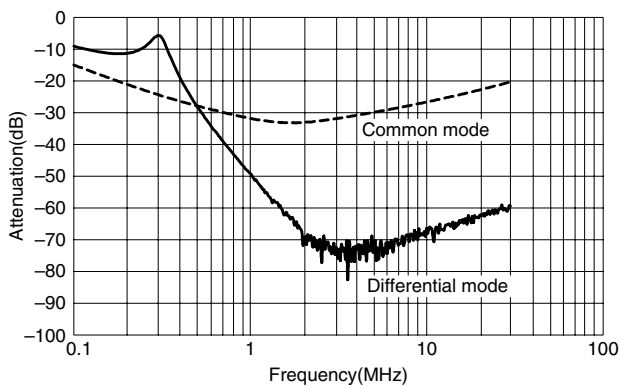
RSEL-2006WL/AL
